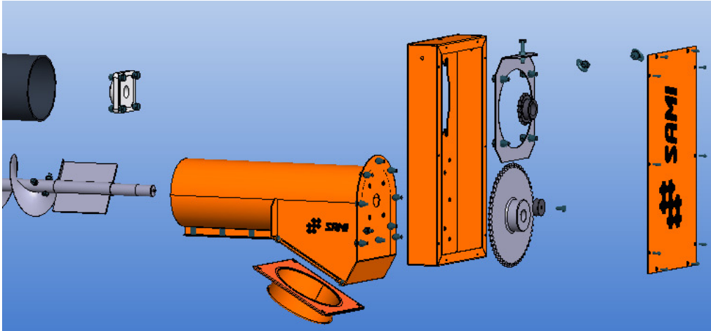
Kuva 2. Purkauspään räjäytyskuva
