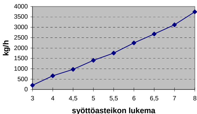
syöttöasteikon lukema kg/h ohralla
