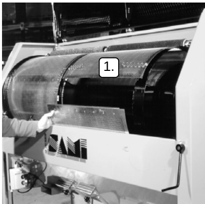
Kuva 12. Seulan kiinnitys.
