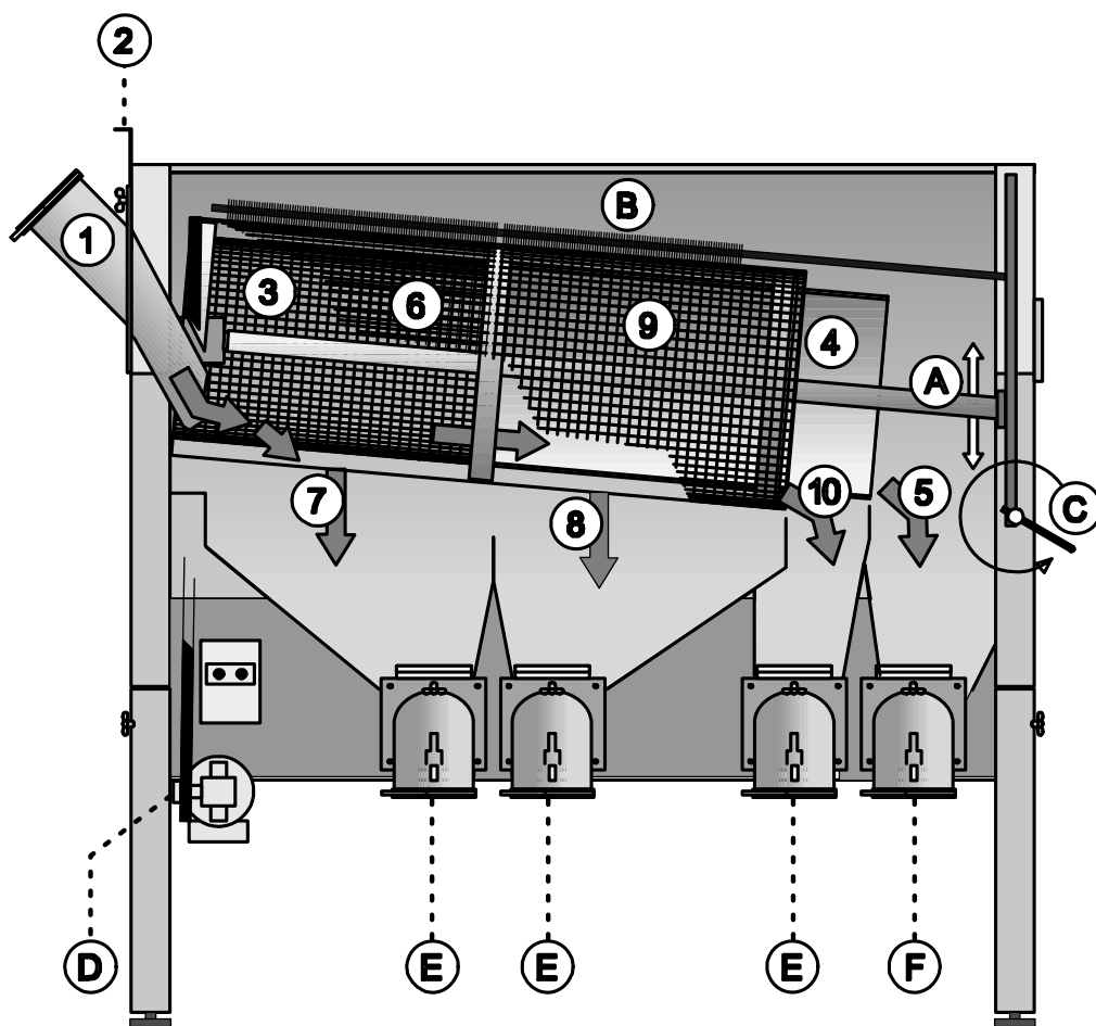
Kuva 3. Lajittimen toimintaperiaatepiirros.
